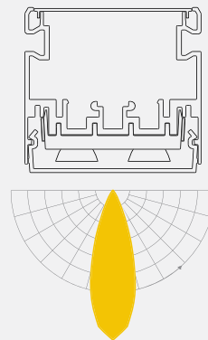
Distribuição intensiva: iluminação em superfícies de trabalho ou em corredores.
