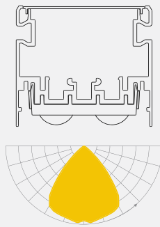
Distribuição média: iluminação otimizada para espaços grandes, corredores e vãos de escada.
