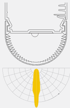
Distribuição intensiva: iluminação de superfícies de trabalho ou em corredores.
