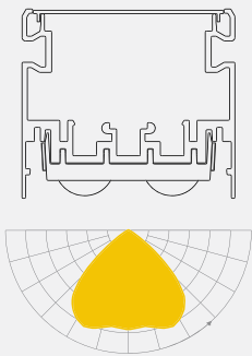
Distribuição extensiva: iluminação uniforme de todo o espaço.
