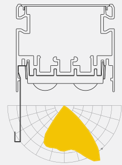
Assimétrica: iluminação de superfícies verticais como postos de trabalho ou expositores com produtos.
