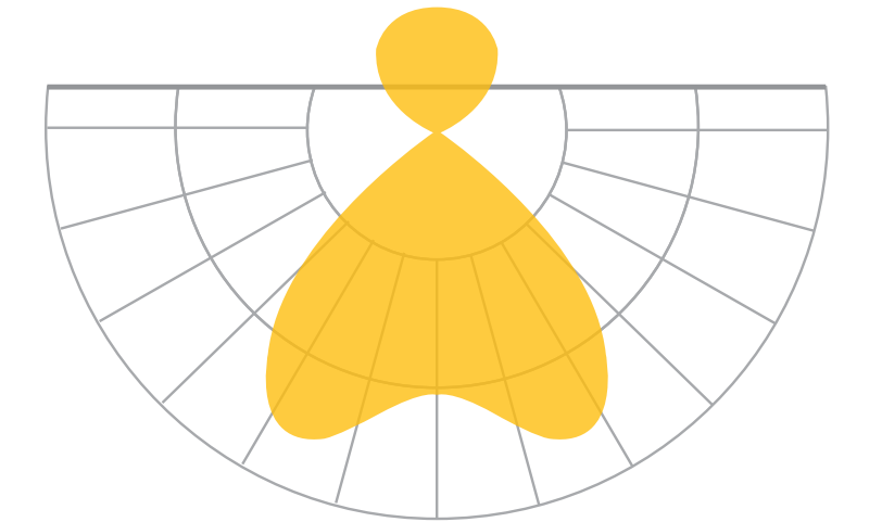
Distribución extensiva con uplight
