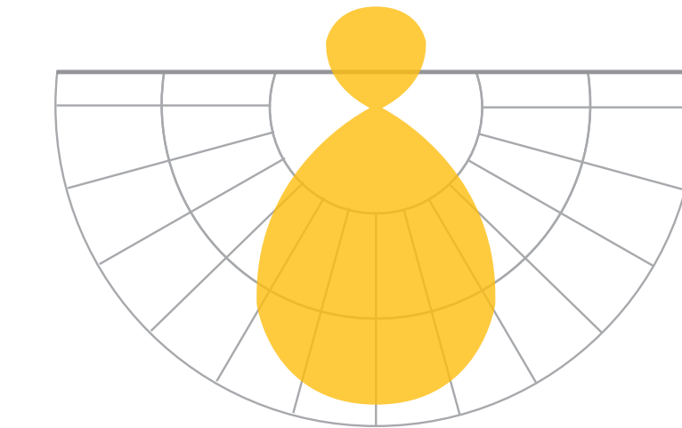
Distribución media con uplight
