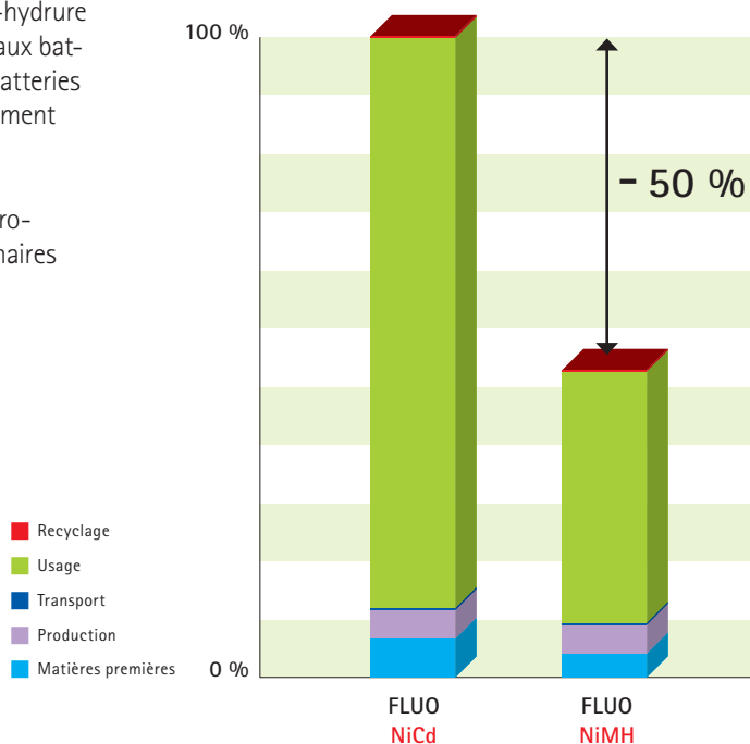
Impact écologique relatif de batteries NiCd par rapport à des batteries NiMH, illustré à l'aide de luminaires non permanents avec une lampe fluorescente de 6W
