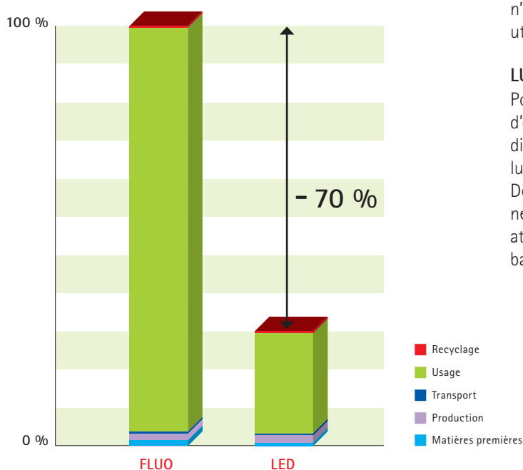
Impact écologique relatif de LED par rapport à des lampes fluorescentes, illustré à l'aide de luminaires permanents pour réseau central
